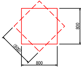
支圧板配置方法 S=1 : 25
