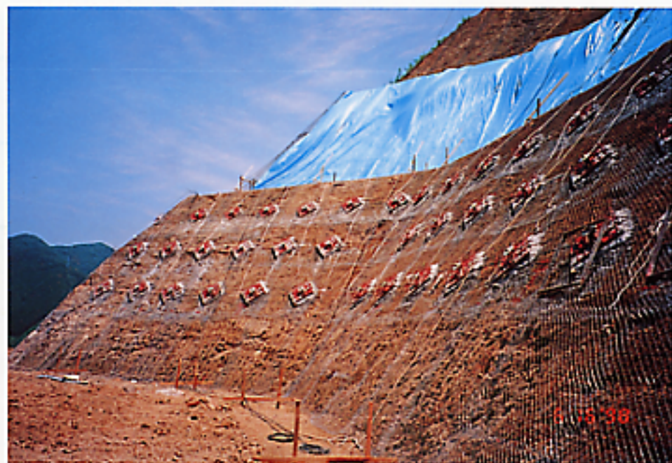
写真-10 支圧板ロックボルト逆巻き工法例
