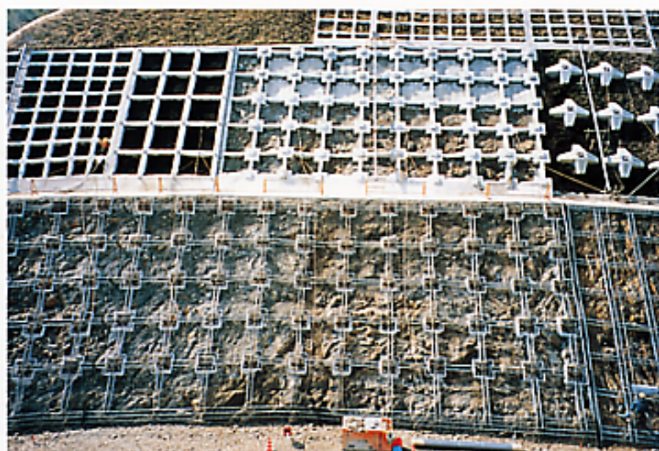
写真-8 支圧板ロックボルト逆巻き工法例
