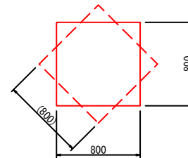
支圧板配置方法 S=1 : 25
