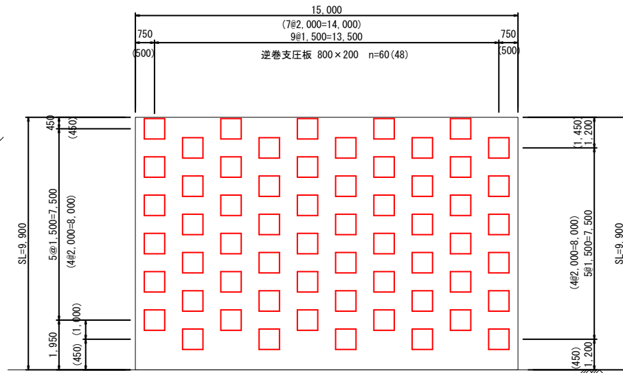
支圧板配置方法 S=1 : 25
