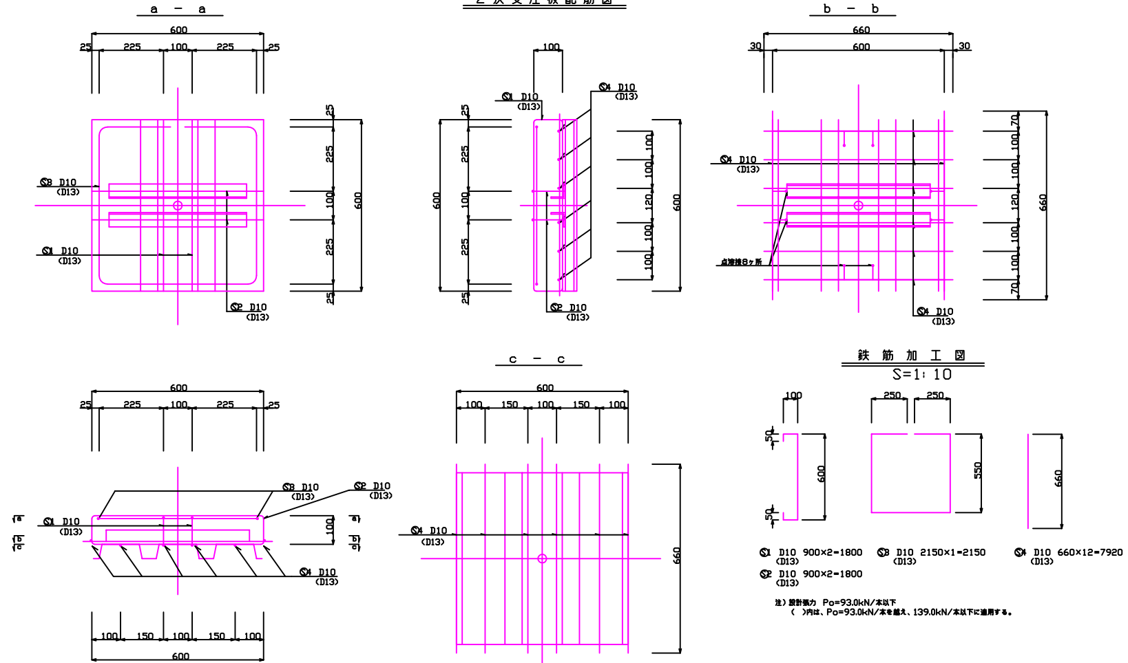
2次支圧板配筋図
