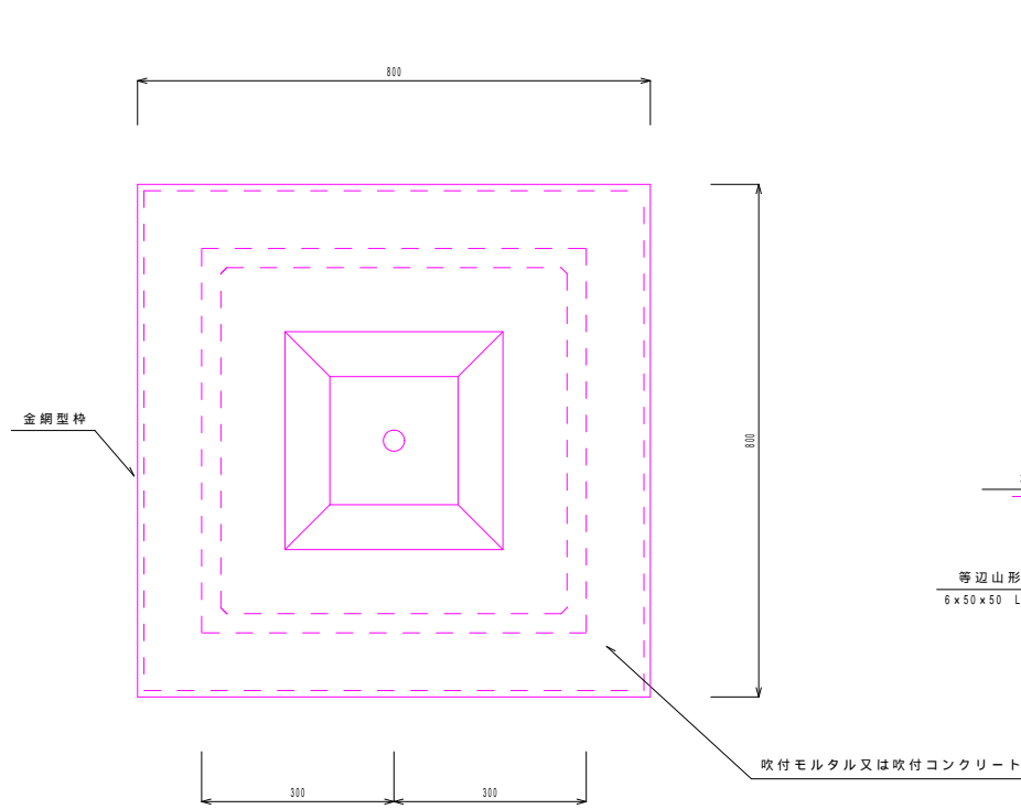
正面図
