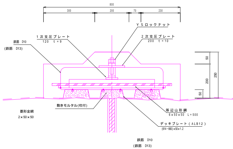
断面図
