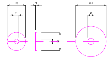
1次支圧プレート 120 t=9
