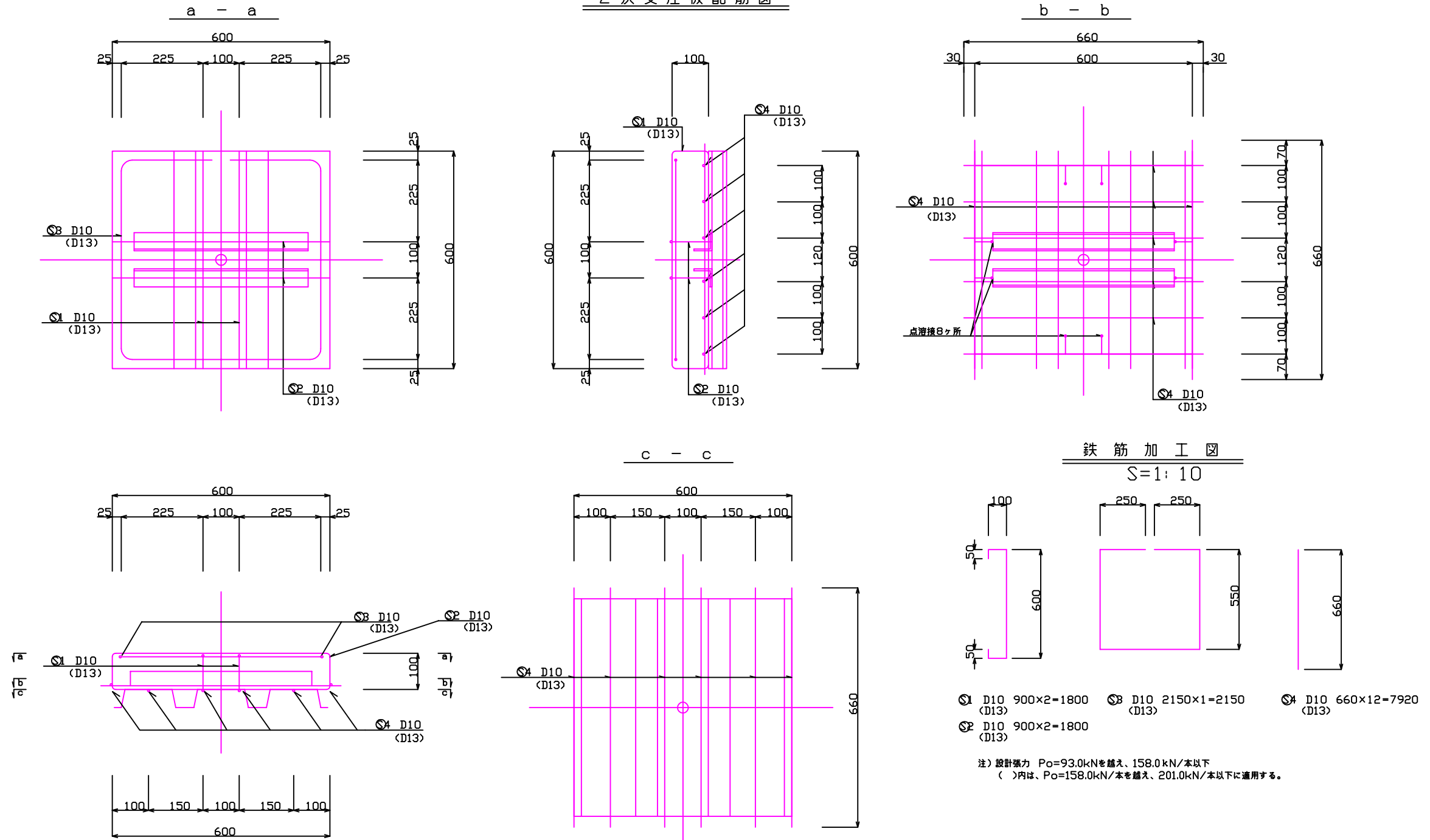
2次支圧板配筋図
