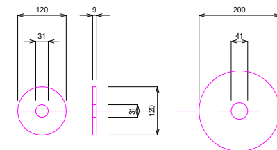
1次支圧プレート 120 t=9
