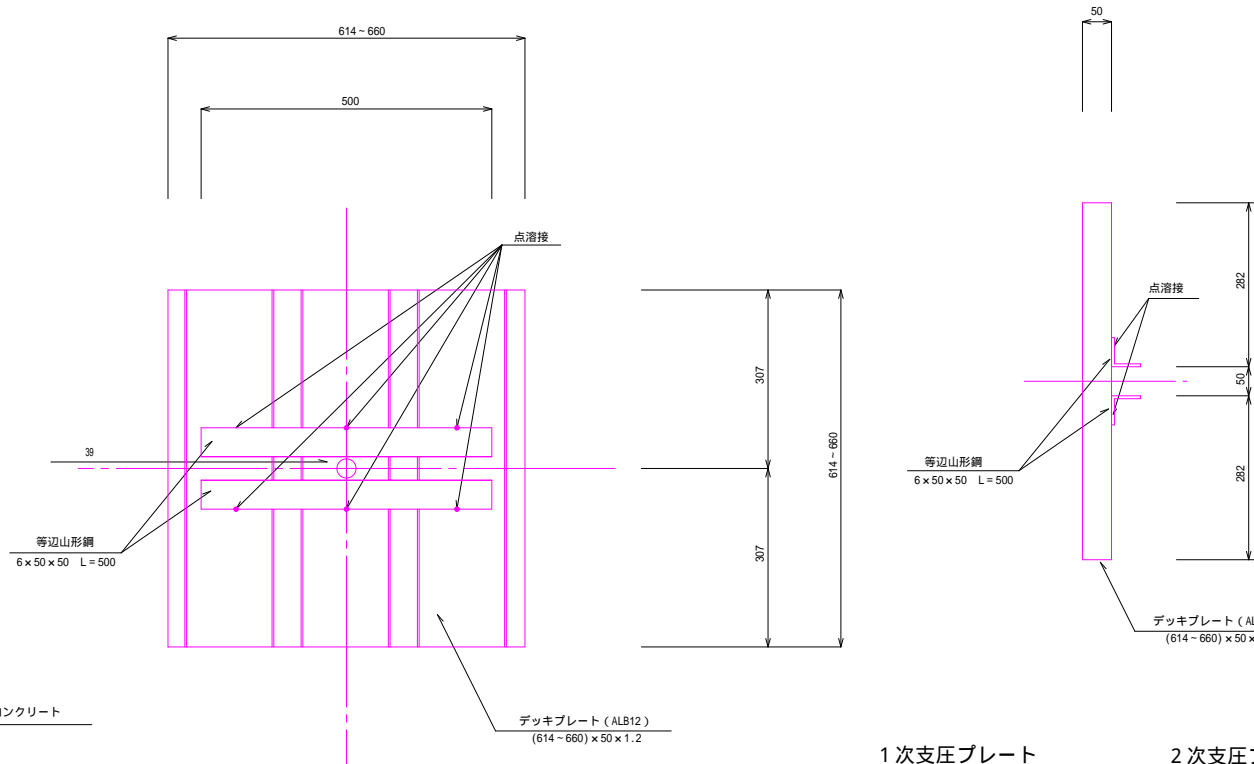
1次支圧プレート 120 t=9
